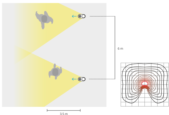
VOIE DE TYPE B - OPTIQUE BF (ASYMÉTRIQUE FRONTALE)
